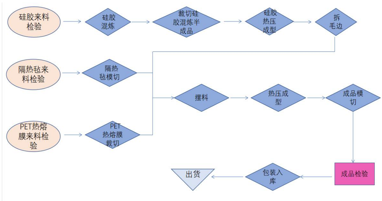
图 2-1 隔热垫生产工艺流程
